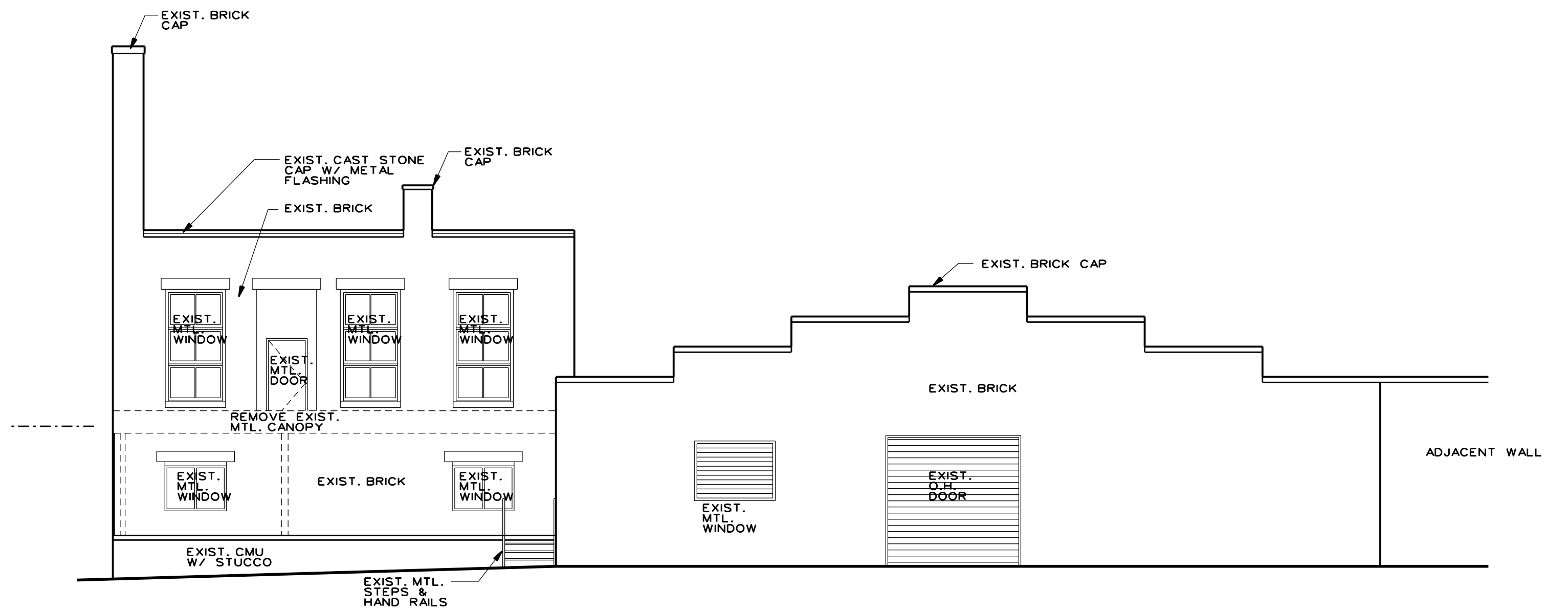
3 A4.2 SOUTH ELEVATION SCALE: 1/8" = 1'-0"
